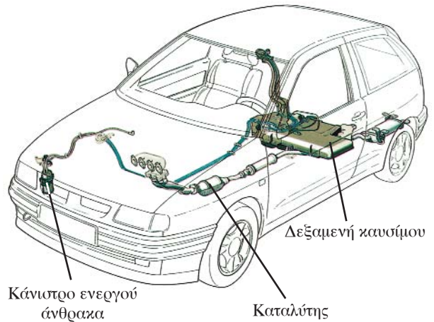
Σχ. 7 Διάταξη αντιρυπαντικών συστημάτων.
