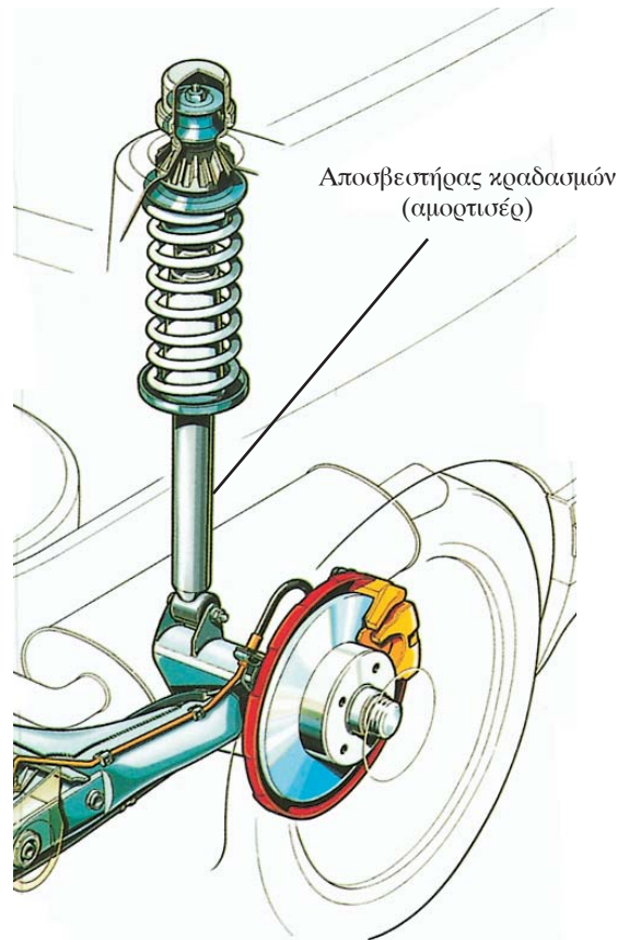
Σχ. 12 Αποσβεστήρας κραδασμών (αμορτισέρ).
