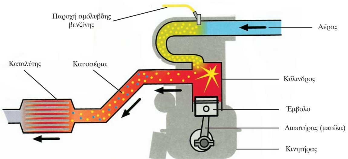
Σχ. 8 Σχηματική παράσταση λειτουργίας κινητήρα με καταλύτη.
