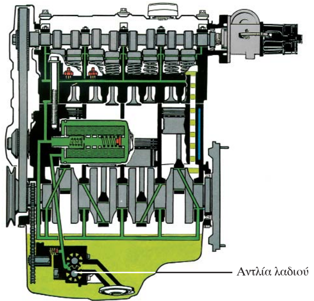
Σχ. 3 Σύστημα λίπανσεως.
